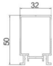
AC45-077 5mm Keel
