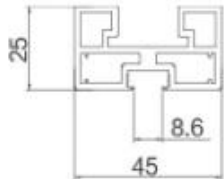
AC45-087 Door Frame
