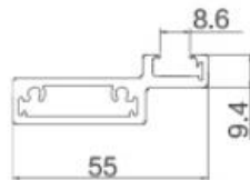
AC45-054A Door Frame
