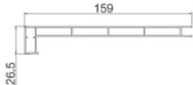
AC45-037 Jamb
