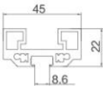
AC45-091 Door Frame
