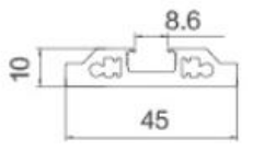
AC45-089 Door Frame
