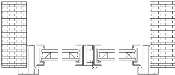
Unequal Double Door
