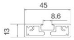
AC45-019 Door Frame
