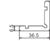
P341 侧板框连接角码
