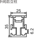
A7388 无线中间后立柱
