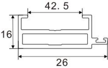
Door Frame Item No.:A-3527 W/T:2.0mm W/M:0.542kg/m
