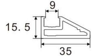
Door Jamb
