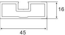
Door Frame Item No.:A-0123 W/T:2.0mm W/M:0.699kg/m
