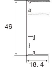
Door Jamb Frame Item No.:A-0186 W/T:1.2mm W/M:0.36kg/m
