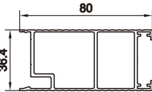
Keel Item No.: A-5028 W/T: 1.2mm W/M: 1.129kg/m
