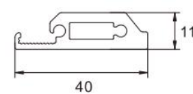
Door Frame Item No.:LJ-8097 W/T:3.0mm W/M:0.606kg/m
