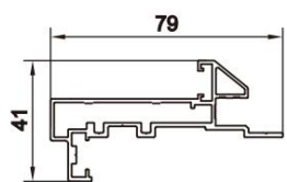
Door Jamb Item No.: A-5004 W/T: 1.2mm W/M: 0.906kg/m
