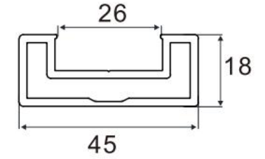
Door Frame Item No.:A-0088 W/T:2.0mm W/M:0.717kg/m
