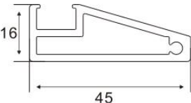
Door Frame Item No.:A-3201 W/T:2.0mm W/M:0.661kg/m
