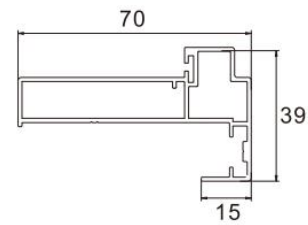
Door Jamb Item No.:LJ-8044 W/T:1.2mm W/M:0.859kg/m
