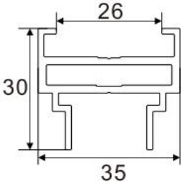
Door Frame Item No.:A-3528 W/T:2.0mm W/M:0.642kg/m
