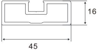
Door Frame Item No.:A-0123 W/T:2.0mm W/M:0.699kg/m
