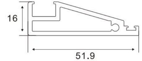
Door Frame Item No.:A-3202 W/T:2.0mm W/M:0.726kg/m
