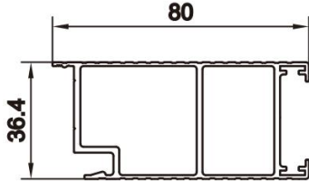
Keel Item No.: A-5025 W/T: 1.2mm W/M: 1.099kg/m
