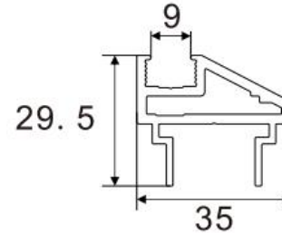
Door Jamb
