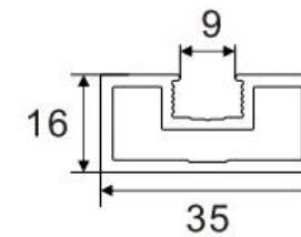
Door Jamb
