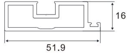
Door Frame Item No.:A-0124 W/T:2.0mm W/M:0.766kg/m
