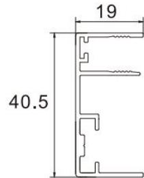
Door Jamb Frame
