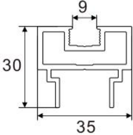
Door Frame Item No.:A-3518 W/T:2.0mm W/M:0.717kg/m
