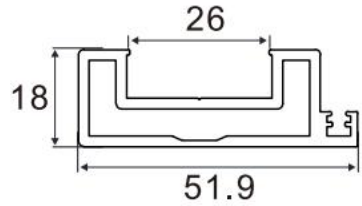
Door Frame Item No.:A-0089 W/T:2.0mm W/M:0.784kg/m
