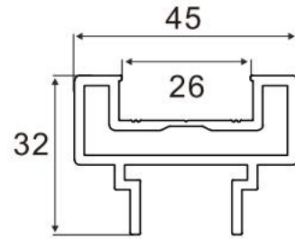
Door Frame Item No.:A-0091 W/T:2.0mm W/M:0.908kg/m
