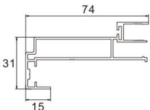
Door Jamb Item No.:LJ-8045 W/T:1.2mm W/M:0.852kg/m
