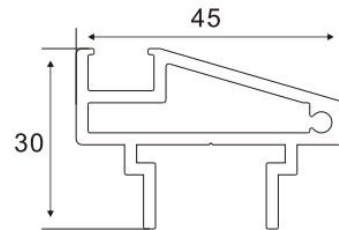
Door Frame Item No.:A-3204 W/T:2.0mm W/M:0.85kg/m
