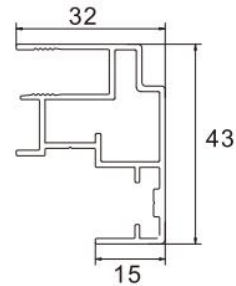
Door Jamb Frame
