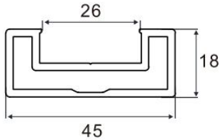
Door Frame Item No.:A-0088 W/T:2.0mm W/M:0.717kg/m
