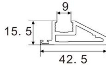
Door Jamb
