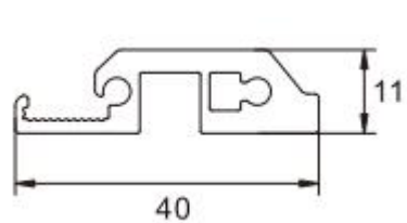
Door Frame
