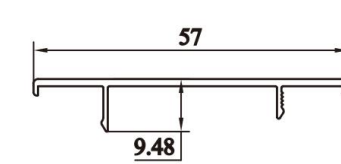
Door Frame Item No.: A-5027 W/T: 1.3mm W/M: 0.24kg/m
