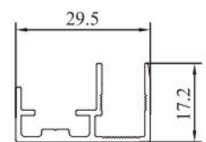
Door Jamb Item No.: A-5003 W/T: 1.2mm W/M: 0.906kg/m
