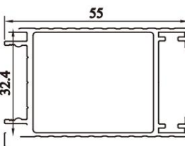
Keel Item No.: A-5010 W/T: 1.2mm W/M: 0.705kg/m
