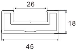
Door Frame Item No.:A-0088 W/T:2.0mm W/M:0.717kg/m
