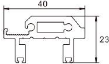
Door Frame
