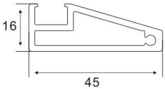
Door Frame Item No.:A-3201 W/T:2.0mm W/M:0.661kg/m
