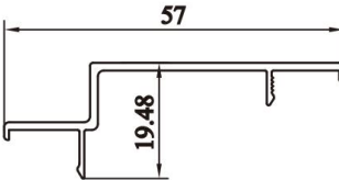
Door Frame Item No.: A-5024 W/T: 1.3mm W/M: 0.276kg/m
