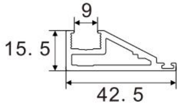
Door Jamb
