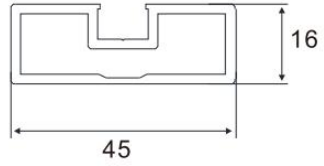
Door Frame Item No.:A-0123 W/T:2.0mm W/M:0.699kg/m
