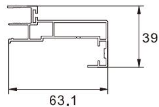
Door Jamb Item No.:LJ-8105 W/T:1.2mm W/M:0.792kg/m
