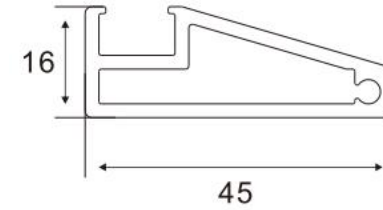
Door Frame Item No.:A-3201 W/T:2.0mm W/M:0.661kg/m
