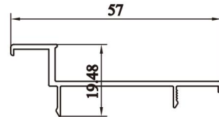
Door Frame Item No.: A-5026 W/T: 1.3mm W/M: 0.287kg/m
