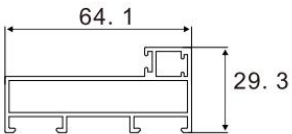
Door Jamb Item No.:A-0115 W/T:1.4mm W/M:0.873kg/m
