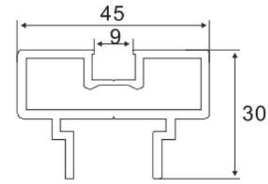
Door Frame Item No.:A-0126 W/T:2.0mm W/M:0.89kg/m
