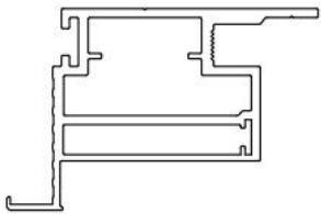
Door Jamb Item No.: A-5015 W/T: 2.0mm W/M: 1.368kg/m
