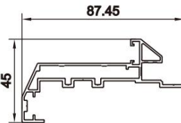
Door Jamb Item No.: A-5005 W/T: 1.2mm W/M: 0.983kg/m
