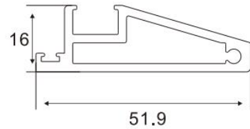
Door Frame Item No.:A-3203 W/T:2.0mm W/M:0.726kg/m
