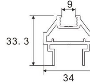
Door Jamb
