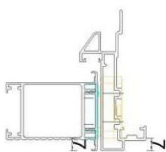
Door Frame Item No.: A-5001 W/T: 1.3mm W/M: 0.199kg/m
