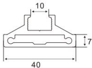
Door Frame
