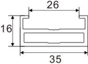
Door Frame Item No.:A-3526 W/T:2.0mm W/M:0.502kg/m
